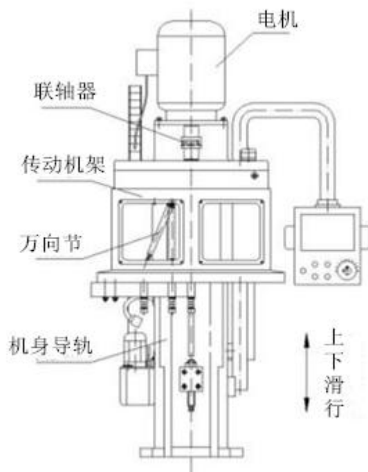
图 12 传动机架
