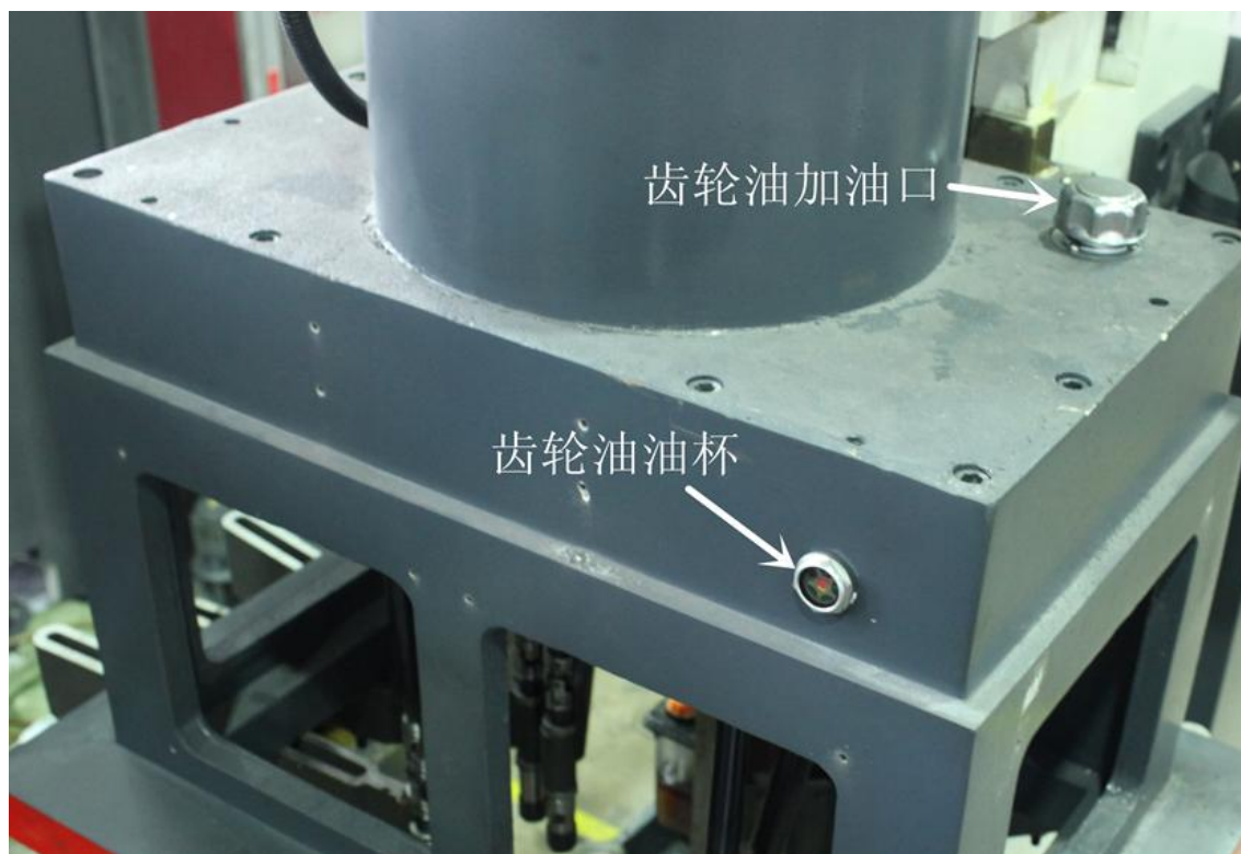
图 7 齿轮油油杯
